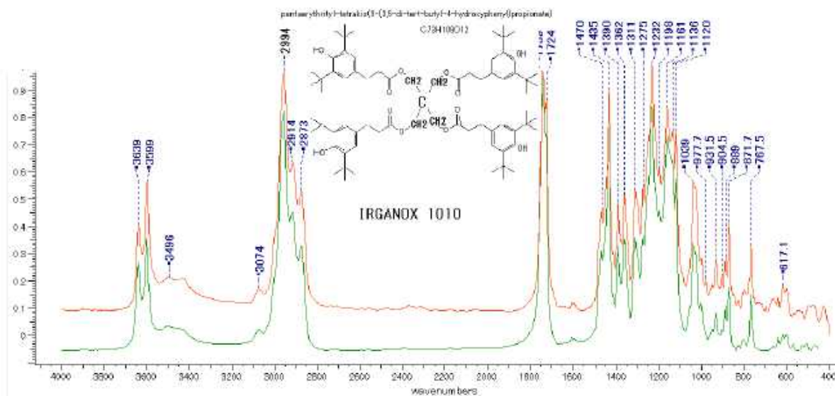
IR-2 Irganox1010 との対比
